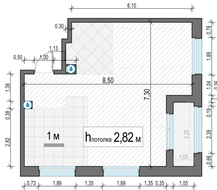
Планировка
