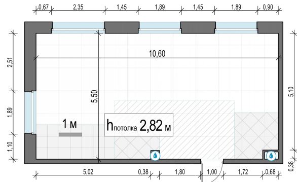
Планировка
