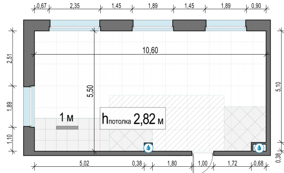
Планировка
