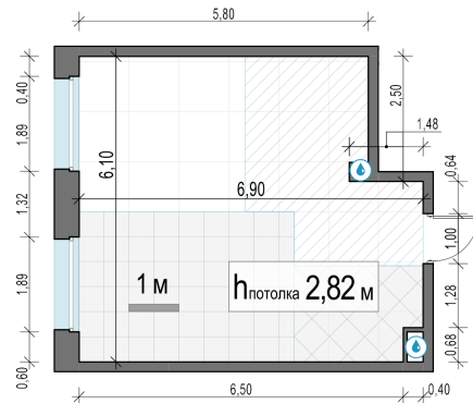
Планировка
