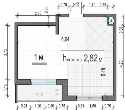
Планировка
