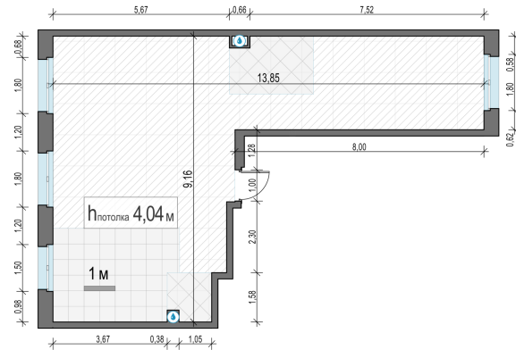
Планировка
