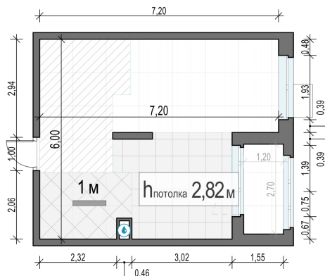
Планировка
