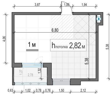
Планировка
