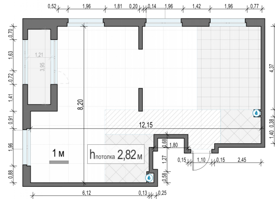
Планировка
