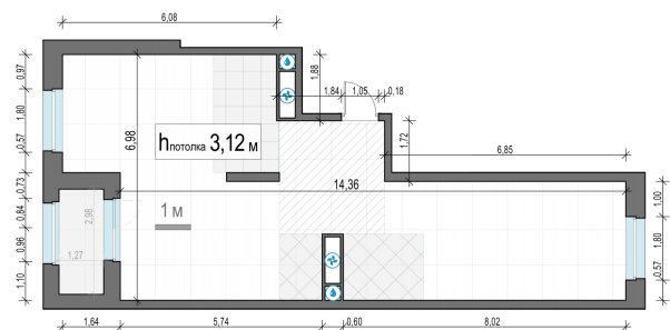
Планировка
