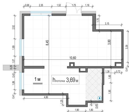
Планировка
