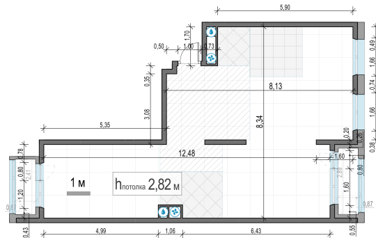
Планировка
