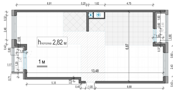
Планировка
