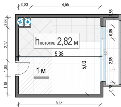
Планировка
