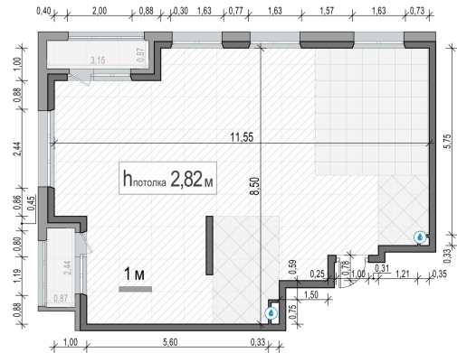
Планировка
