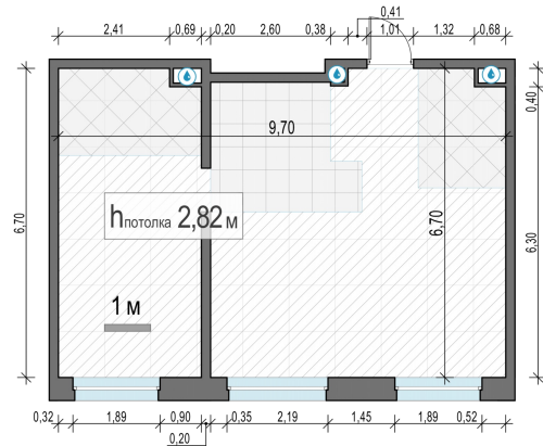
Планировка
