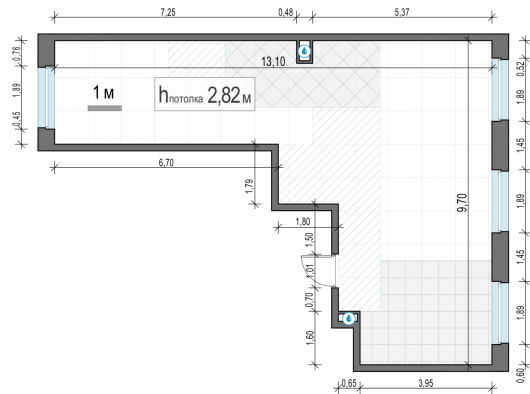
Планировка
