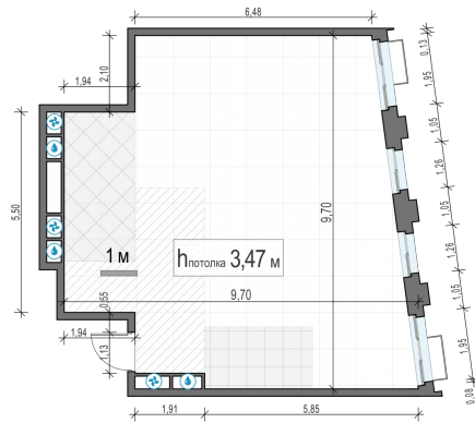
Планировка
