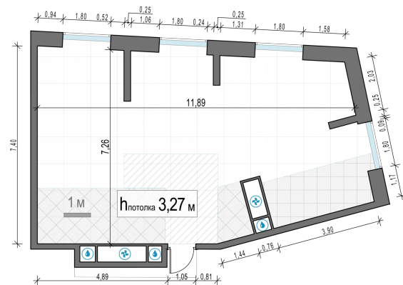
Планировка
