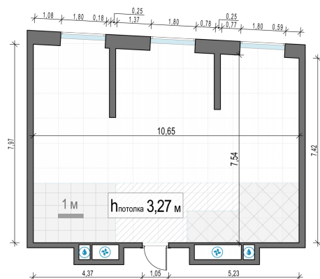
Планировка
